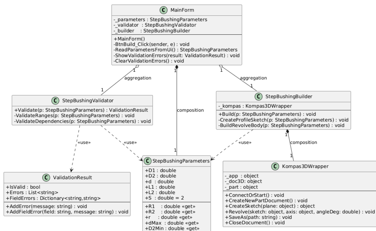
Рисунок 3.1 – UML-диаграмма классов плагина «Ступенчатая втулка»
