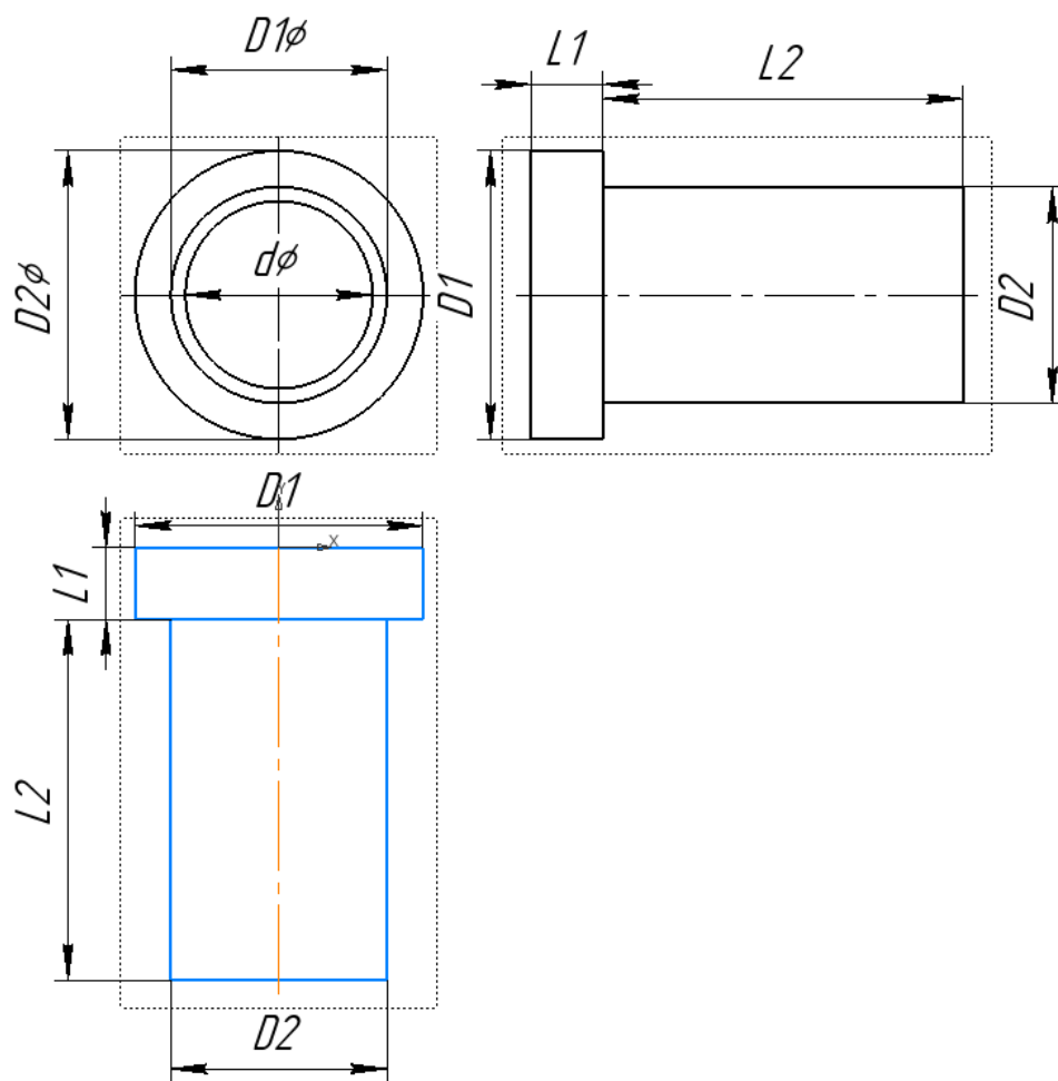
Рисунок 2.1 — Модель ступенчатой втулки
